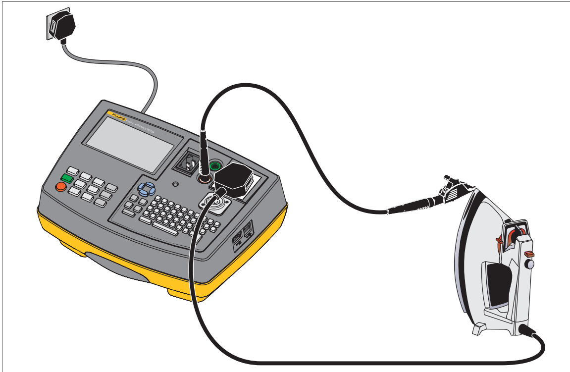
Afbeelding 7. Aansluitingen voor aanraakstroomtest
