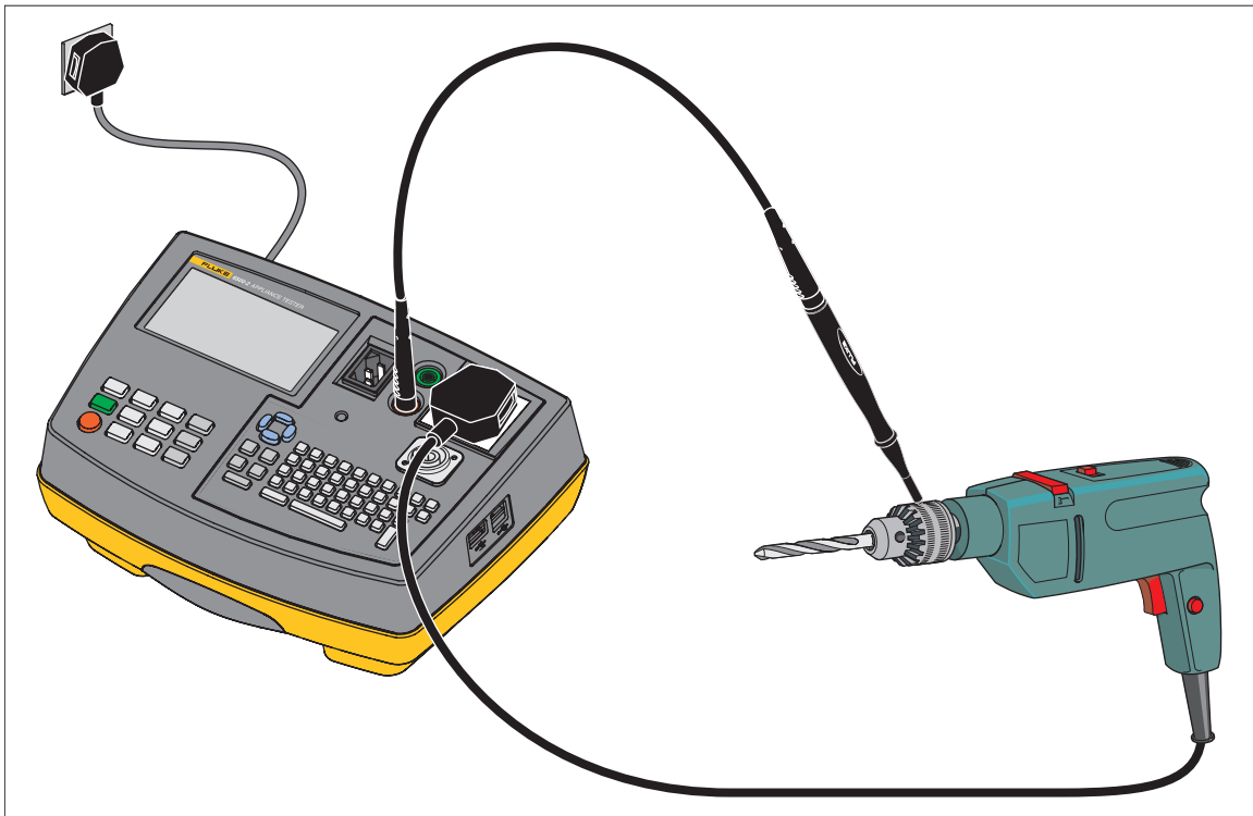
Afbeelding 6. Aansluitingen voor vervangende-lekstroomtest voor klasse II
