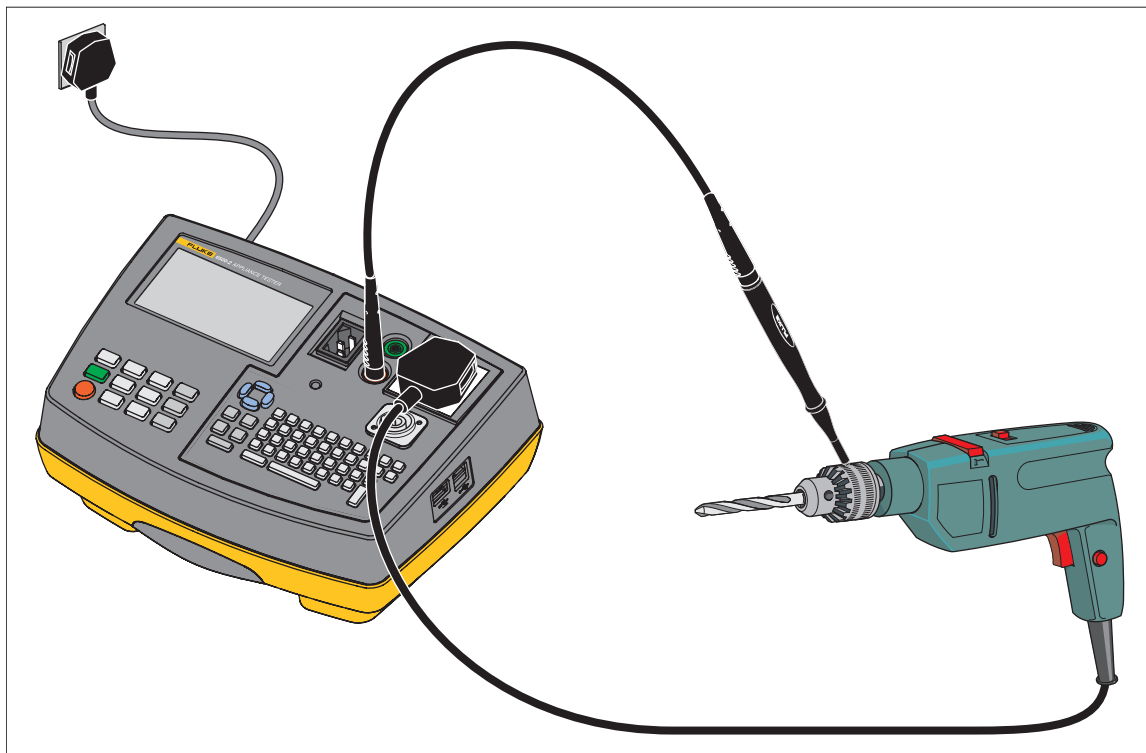
Afbeelding 4. Aansluitingen voor isolatietest voor klasse II
